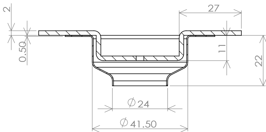
断面図 A-A
