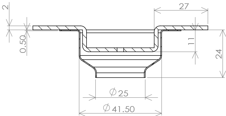
断面図 A-A
