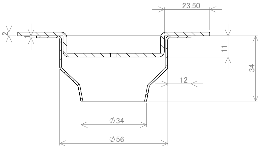
断面図 A-A
